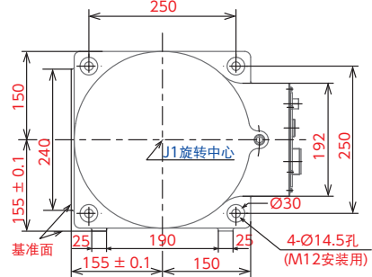
底座安装尺寸 (B-B视图)
