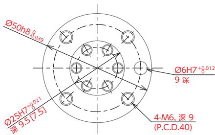
工具安装面详图 (箭头所示A)
